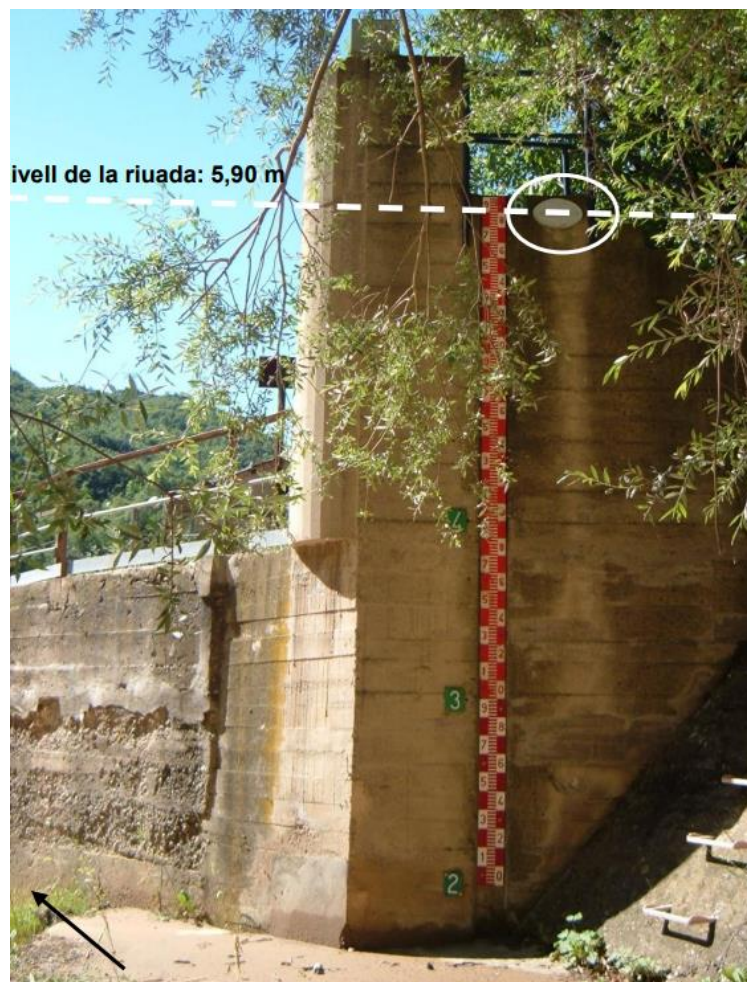
Limnimarca del riu Llobregat 12-10-1907 Estació d'aforament EA-078 GUARDIOLA DE BERGADA - BERGADA
